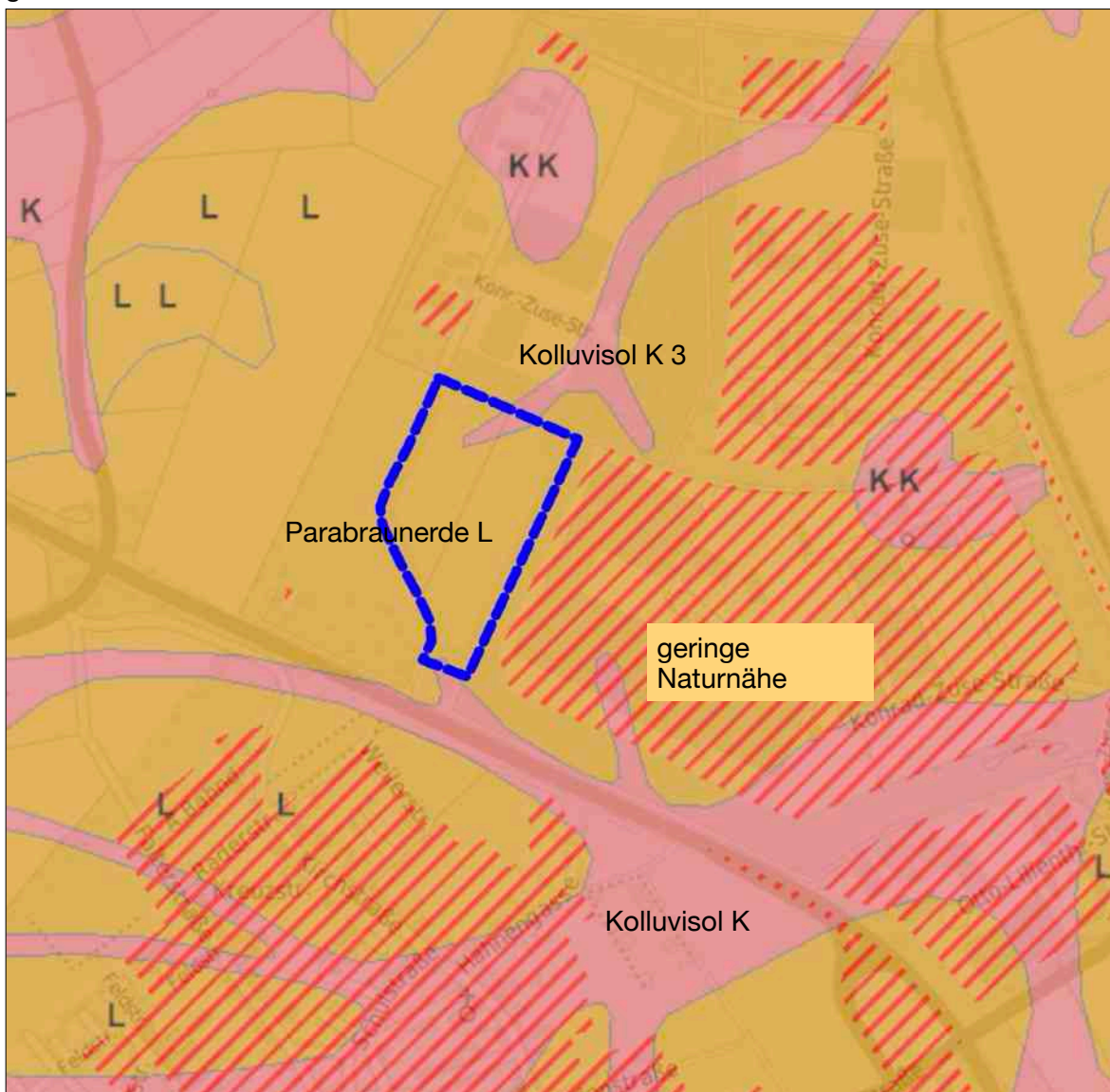
Abb. 20: Auszug aus der Bodenkarte BDK 50 (Quelle: https://geoportal.staedteregion-aachen.de )
