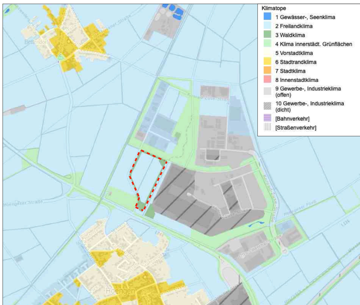
Abb. 22: Auszug aus der Klimatopkarte NRW 10
